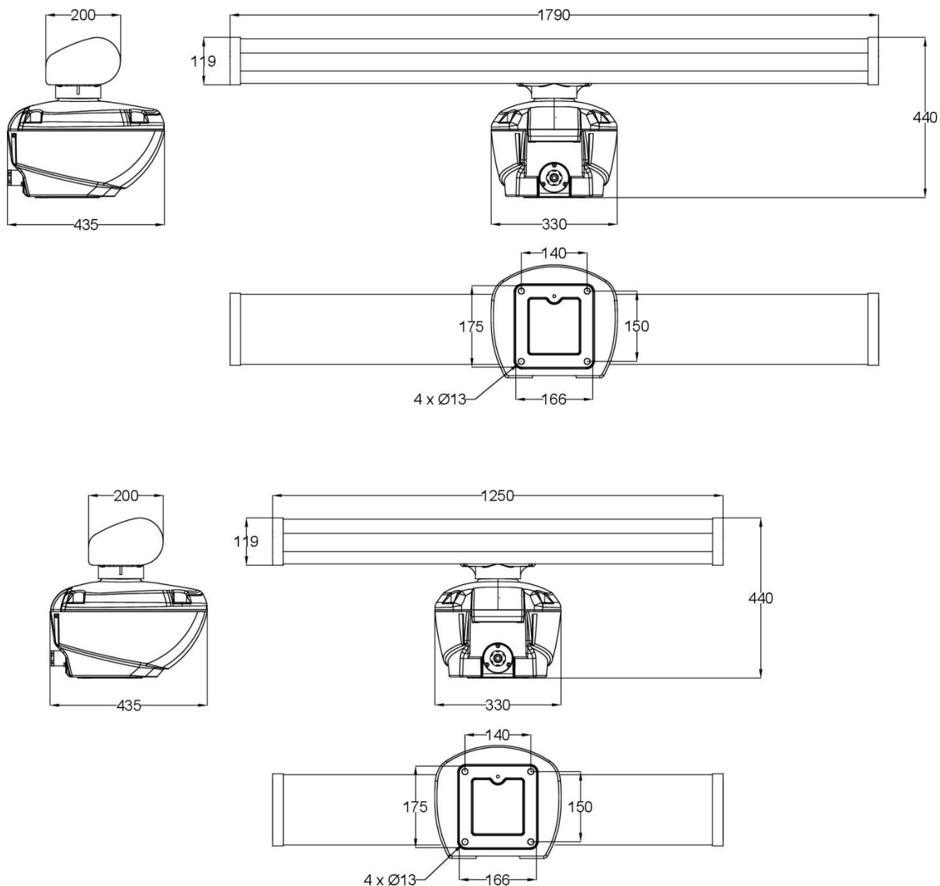
Габаритные размеры антенны «АМ18» и антенны «АМ12»
